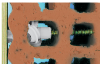
Optimální zauzlení v dutinových tvárnících
